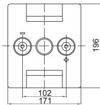
F10 TERMINAL
